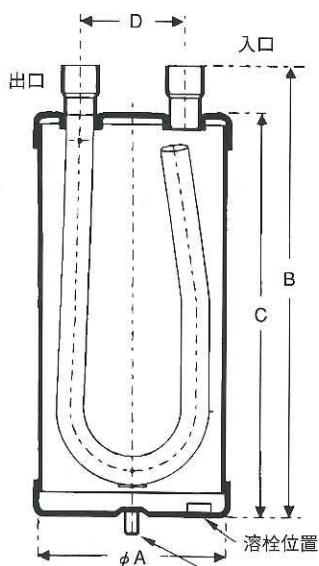
底部取付ねじ 3/8-16UNC (ナット付)
